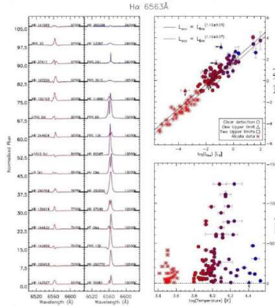
Şəkil 1. HAe və HBe ulduzlarının xətt profilləri; hər sütun aşağıdan yuxarıya doğru artan temperatur ardıcılığındadır. H \alpha xəttin ekvivalent eninin ulduzun temperaturundan asılılığı.
